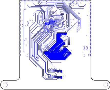
Bottom Layer (Scale 1:1.43)
