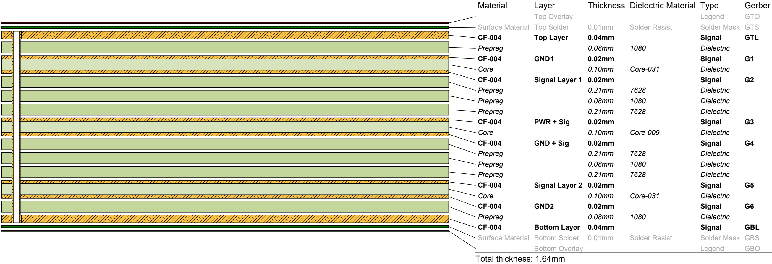
Layer Stack Legend
