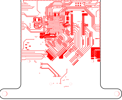
Top Layer (Scale 1:1.43)
