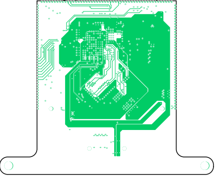
PWR + Sig (Scale 1:1.43)
